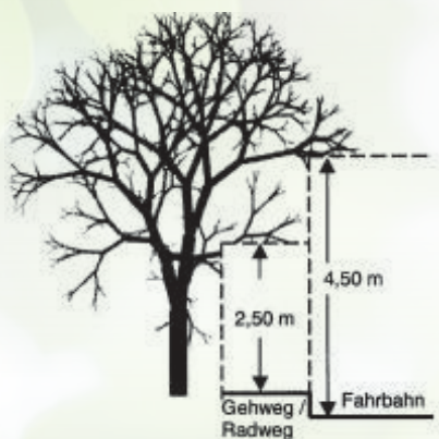
Frei zu haltendes Lichtraumprofil
